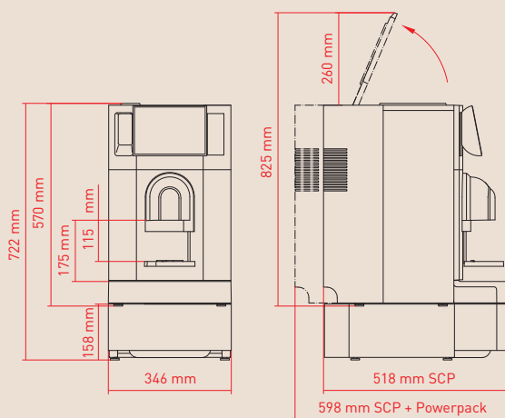
Schaerer Coffee Prime mit Powerpack und Kühleinheit unter der Maschine
