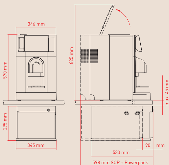
Kühleinheit unter der Maschine und unter der Theke
